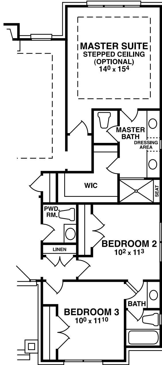
OPTIONAL 3 BEDROOM PLAN
